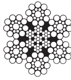
6 x 19 Seale (1+9+9) + SES
