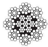
8 x 19 Seale (1+9+9) + SES
